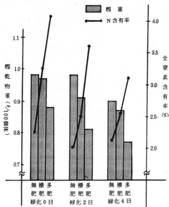
第2図 処理と乾物重および全窒素含有率との関係
