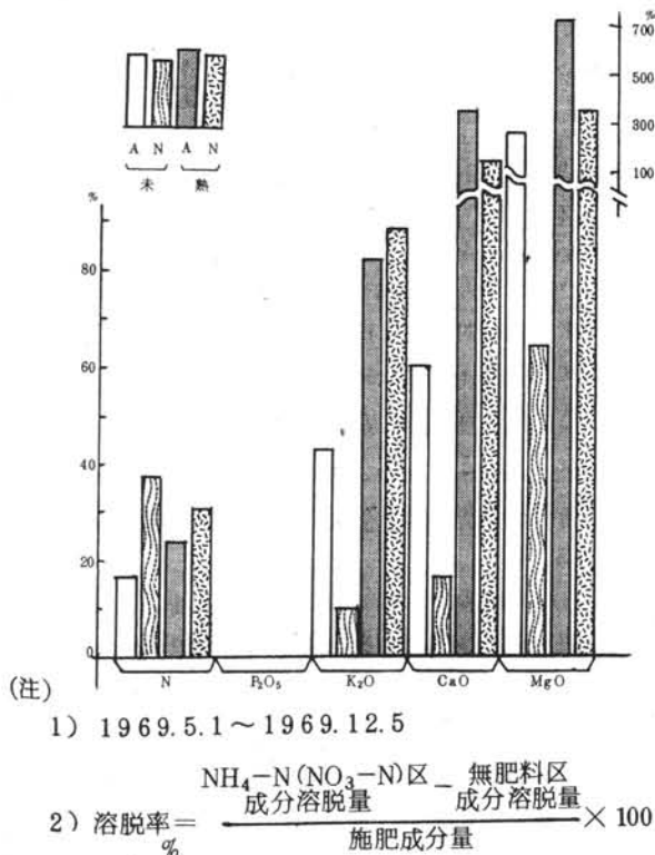
図10 各成分の溶脱率
