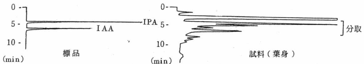
第1図 Nucleosil 5 N (CH 3 ) 2 カラムによるオーキシンのクロマトグラム
