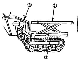
①荷台 ②油圧シリンダー ③開放レバー
