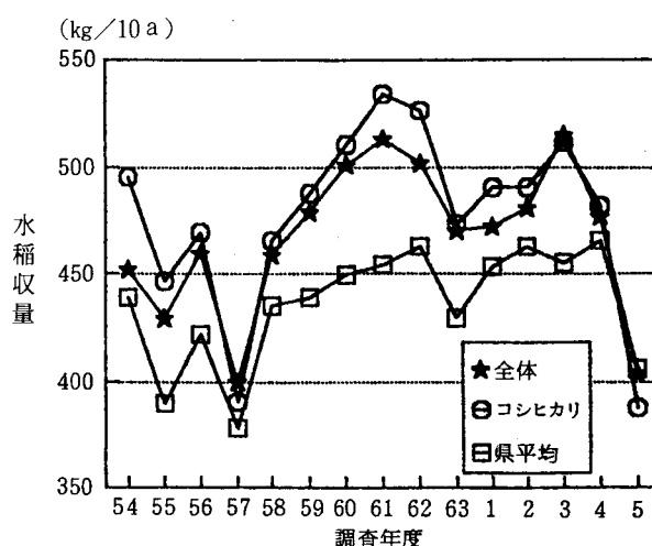
図2 定点における水稻収量の変化
